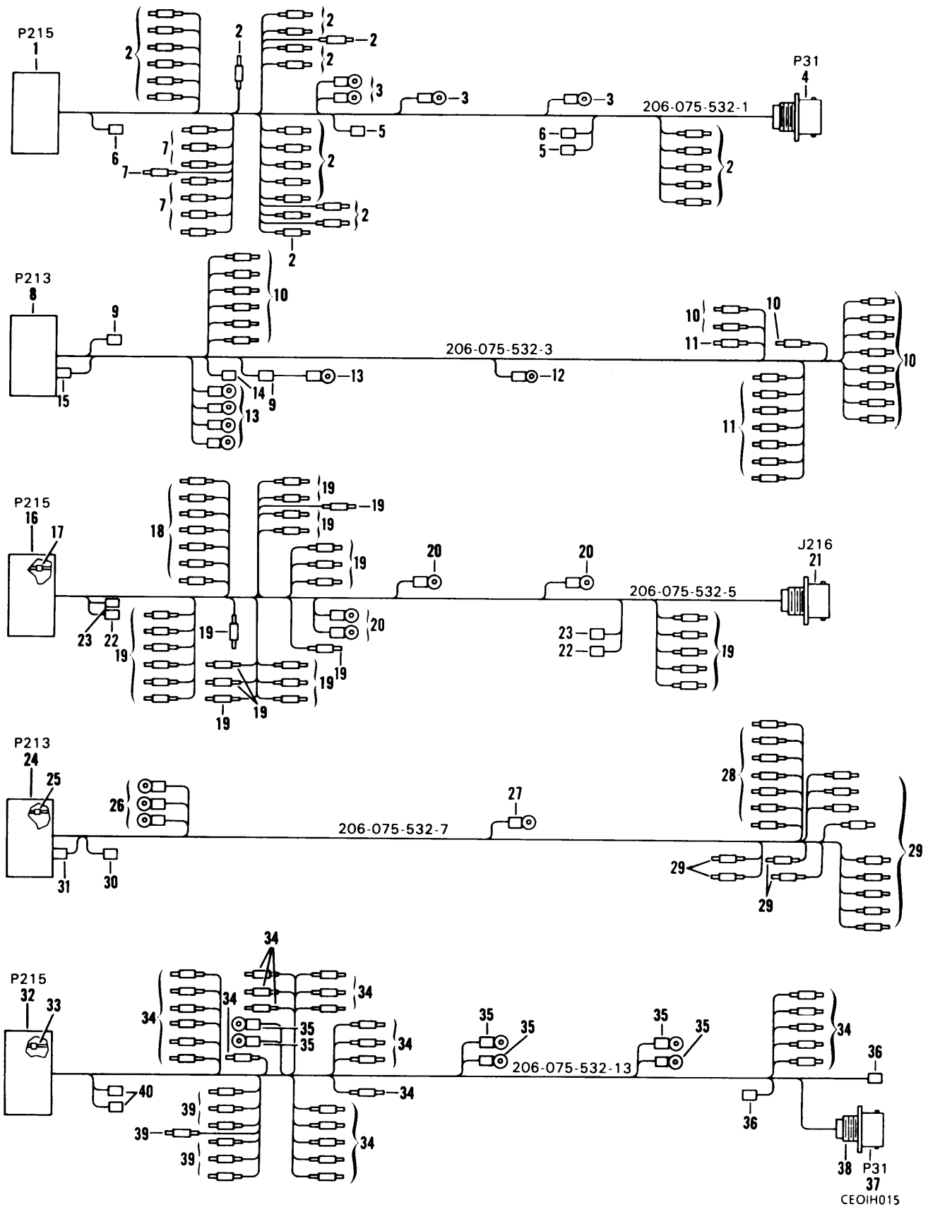
Figure 9. Cable Assemblies (206-075-532-1, 206-075-532-3, 206-075-532-5, 206-075-532-7, 206-075-532-13).
